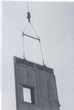
◀パネルの吊り上げ
