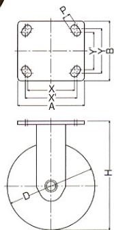
500BPR-CR 150mm
