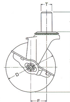
315EK-UR 100mm
